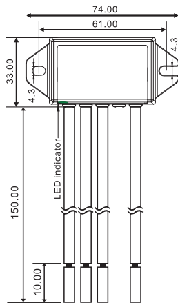
ZP-LED-P10B(5L)
