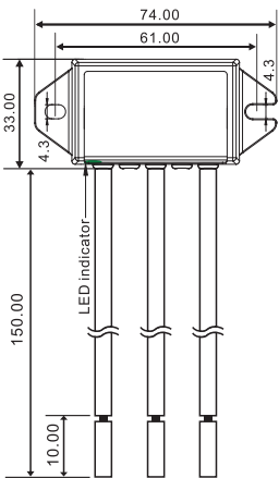
ZP-LED-P10B(3L)
