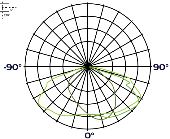
Luminaire
