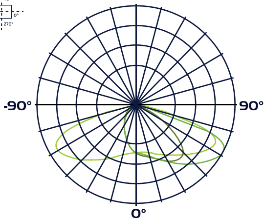
Luminaire
